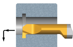
Zapichování
