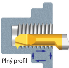
Závitování
